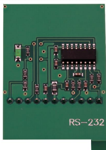
Рисунок 8. Плата преобразователя уровня RS-232
