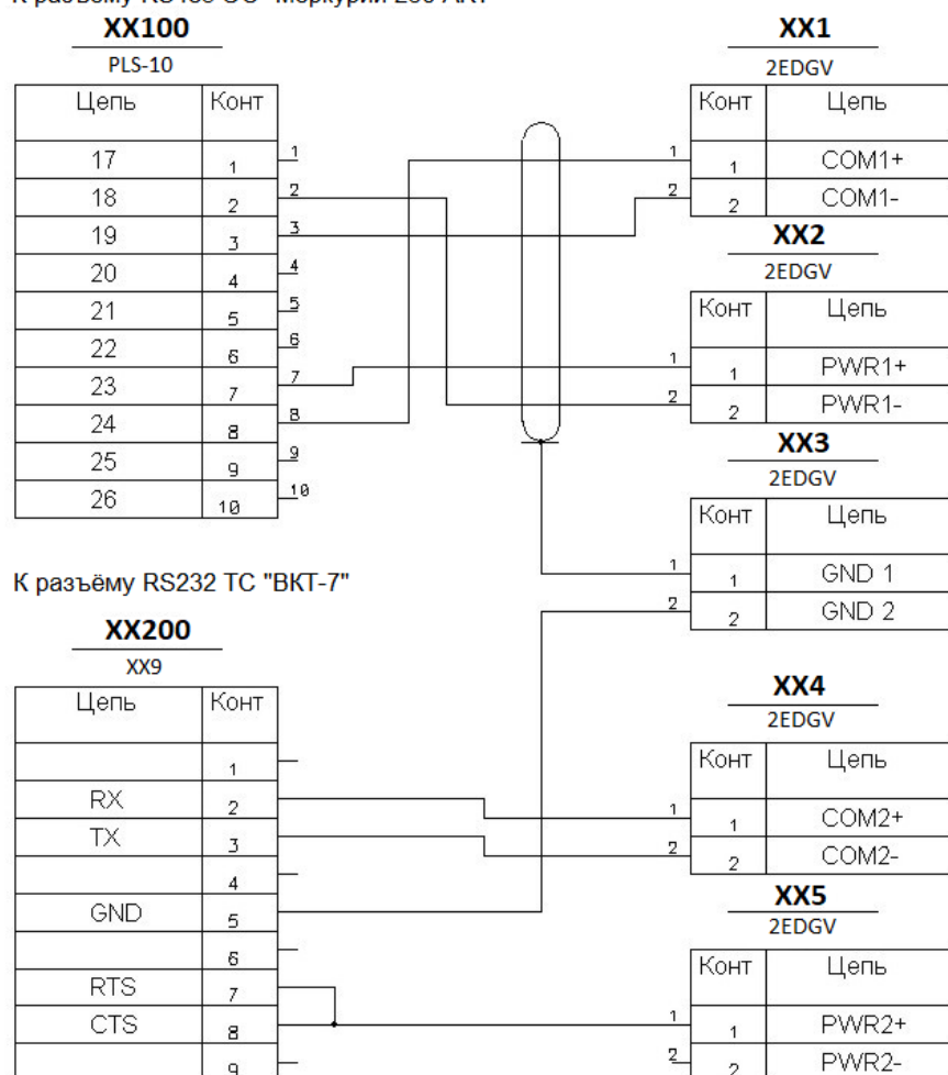
Рисунок 11. Схема подключения счетчиков по RS-485 и RS-232
