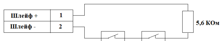
Рисунок 5. Подключение извещателей с нормально замкнутыми контактами
