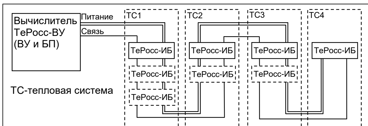
Рисунок 3.1 – Структурная схема прибора ТеРосс-ТМ
