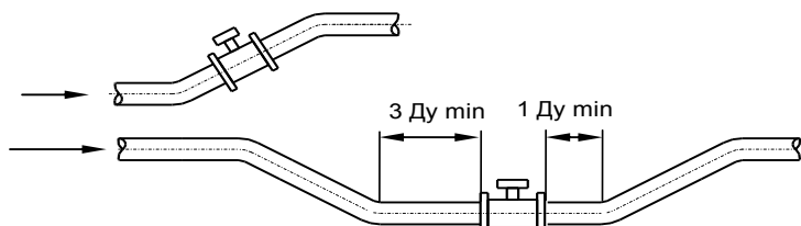
Рис. В.2 Примеры горизонтальной установки ППР
