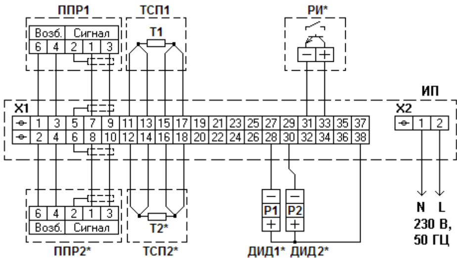
Рис. Е.1 Схема электрических соединений теплосчётчика ТЭPM-02-6-Х. Примечание. * - опционально, в зависимости от исполнения.
