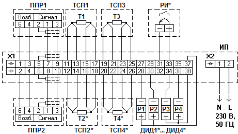
Рис. Е.2 Схема электрических соединений теплосчётчика ТЭPM-02-7-Х. Примечание. * - опционально, в зависимости от исполнения.
