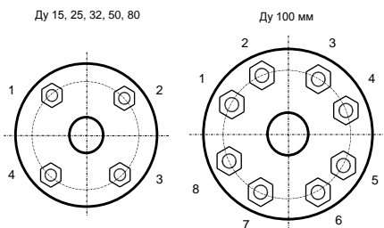
Последовательность затяжки гаек: 1-3-4-2 Последовательность затяжки гаек: 1-5-7-3-2-6-8-4
