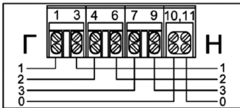
Рисунок В.5 – Тип корпуса S31 исполнение А
