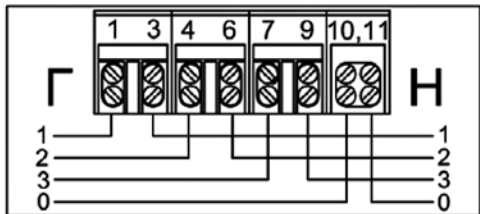
Рисунок В.7 – Тип корпуса S31 исполнение R2
