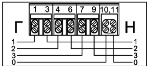
Рисунок В.1 – Тип корпуса R33 исполнение А
