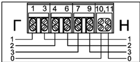
Рисунок В.8 – Тип корпуса S31 исполнение R2S
