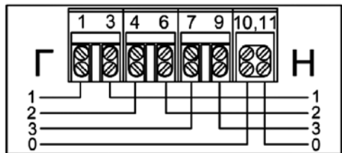
Рисунок В.4 – Тип корпуса S31 исполнения PS, R1S
