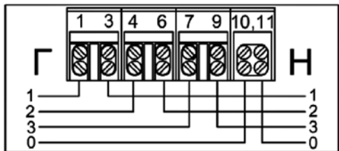
Рисунок В.3 – Тип корпуса S31 исполнения P, R1
