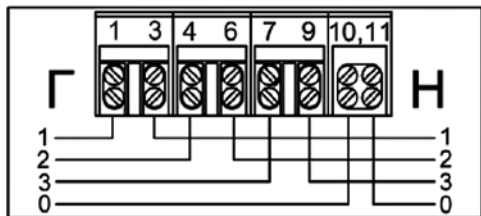
Рисунок В.2 – Тип корпуса R33 исполнение AS
